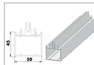
Sparren 45 mm
