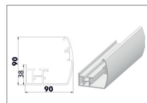
Rinne 90 mm
