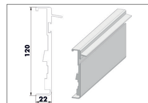
Wandanschluss 120 mm
